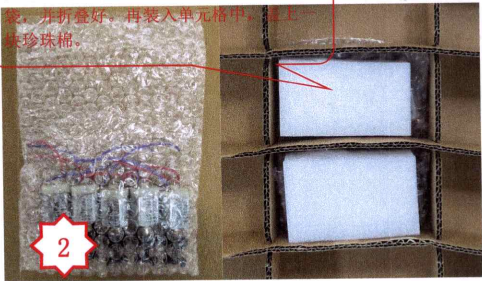
图二，将 1PCS PA2616 如图装入气泡袋，并折叠好。再装入单元格中。（每个单元格装入 1 袋，上面需盖 1 块珍珠棉）
