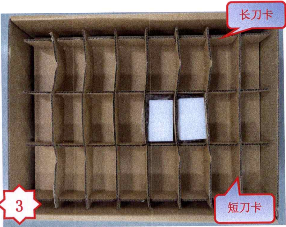
图三，将 PA2616 按照每层 120PCS，每箱 3 层的方式进行包装，同时在底层和每层的顶部放一块隔板，共 3 块隔板。
